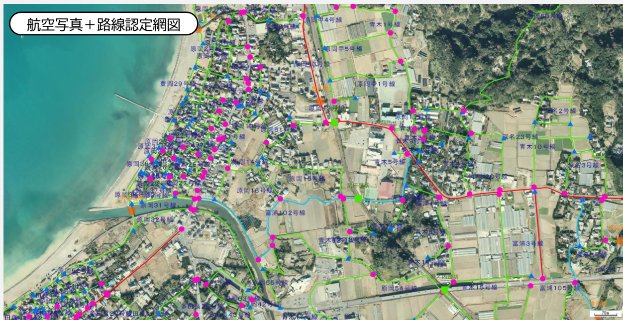
道路台帳図
