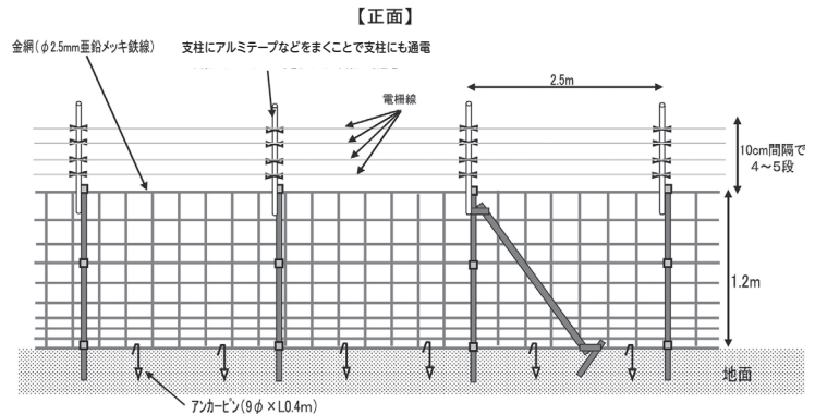
サル用複合柵(金網柵+電気柵)設置例
