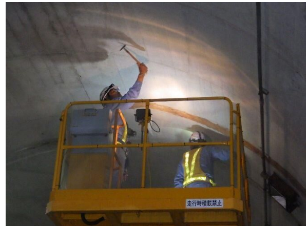
写真 3.2 近接目視点検・打音調査
